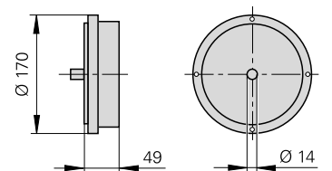
ROD 780, ROD 880
